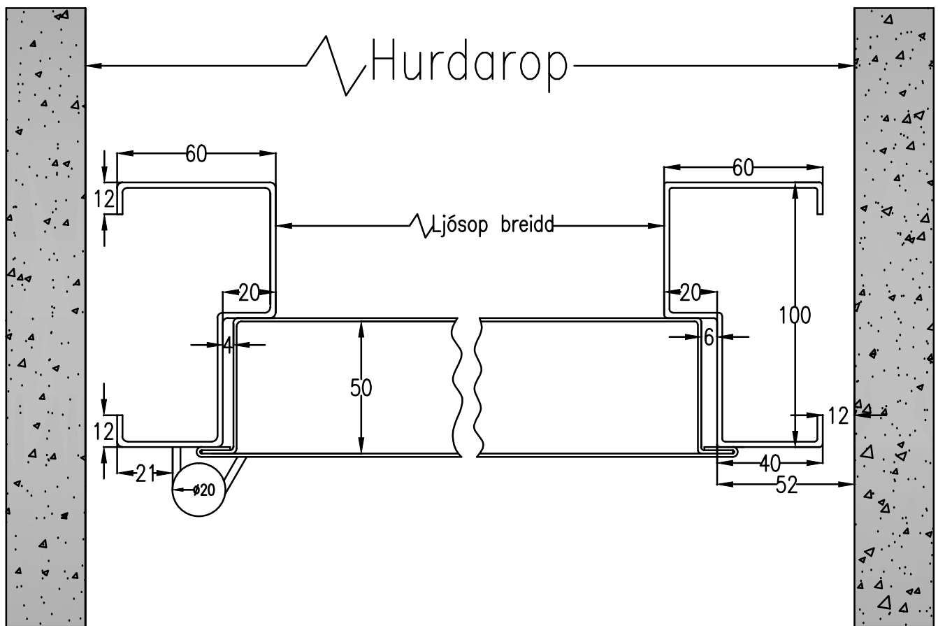
Þversnið, einföld hurð, karmur B
