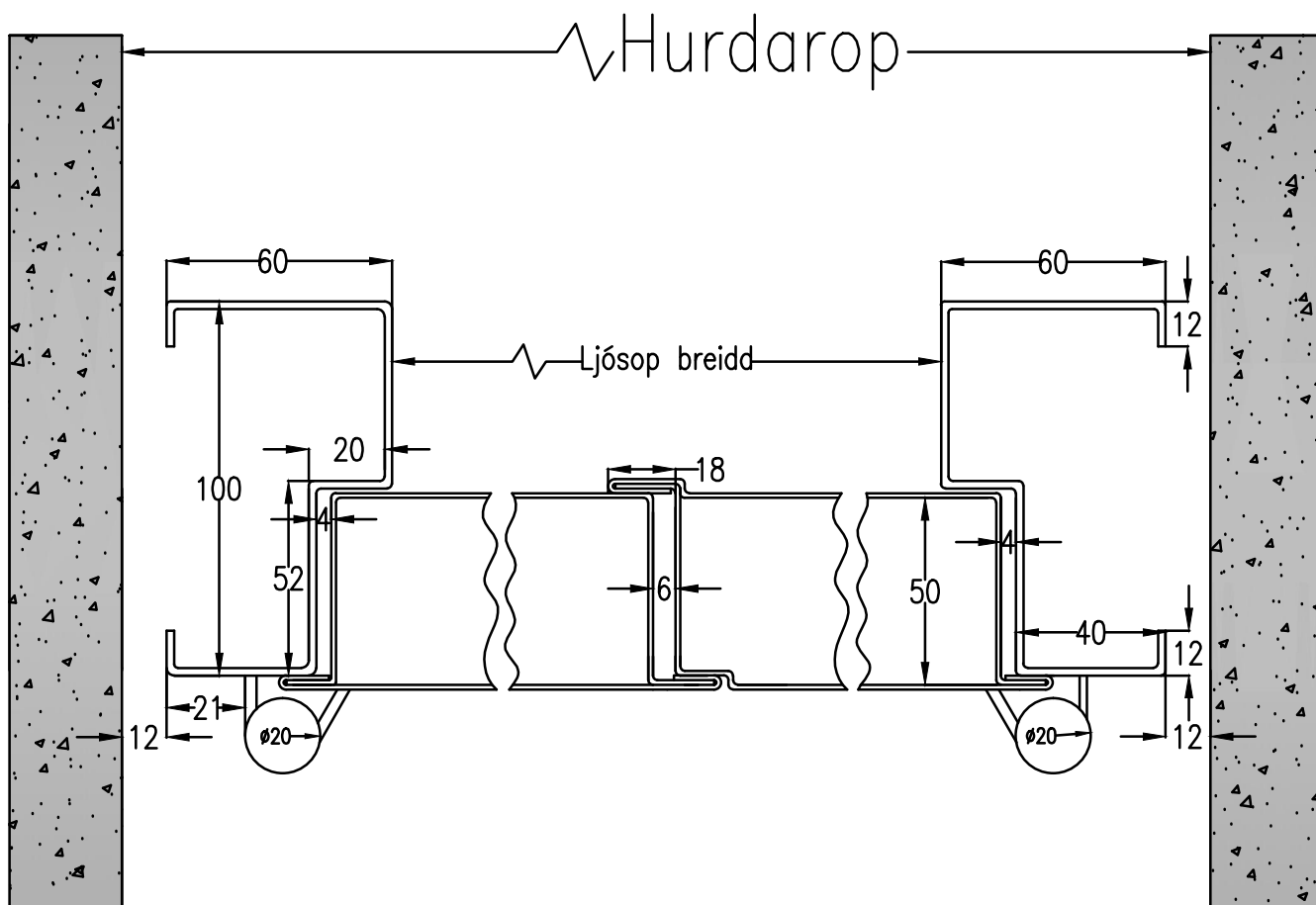
Þversnið, tvöföld hurð, karmur B
